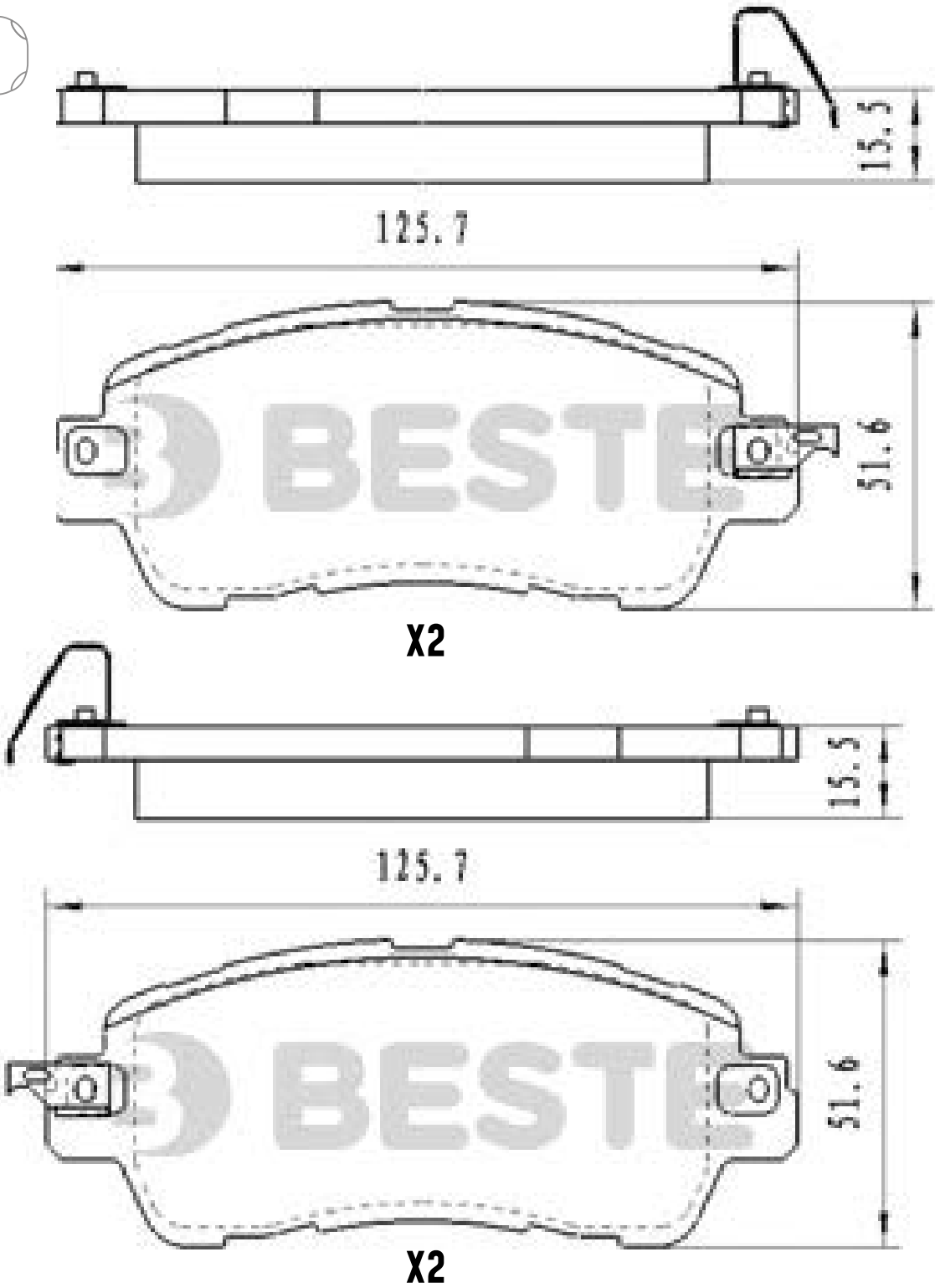
EJE DELANTERO
