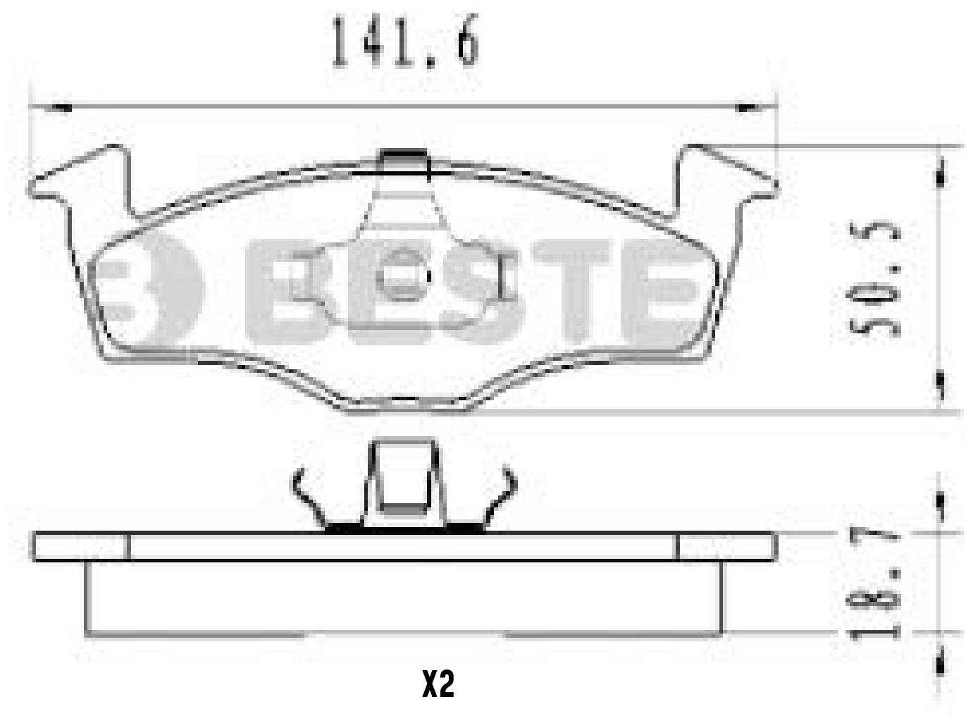
EJE DELANTERO
